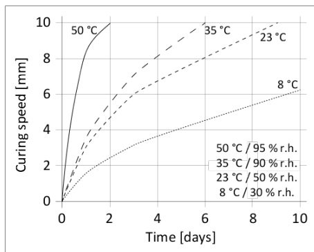
Διάγραμμα 1: Ταχύτητα ωρίμανσης σιλικονών Sikasil® SG-20
