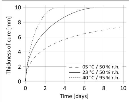
Διάγραμμα 1: Ταχύτητα ωρίμανσης Sikasil® WS-605 S
