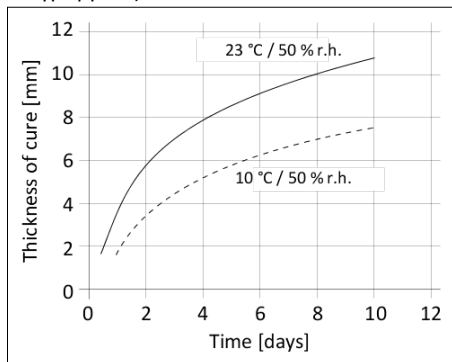
Διάγραμμα 1: Αντίδραση ωρίμανσης για το Sikaflex®-291i.
